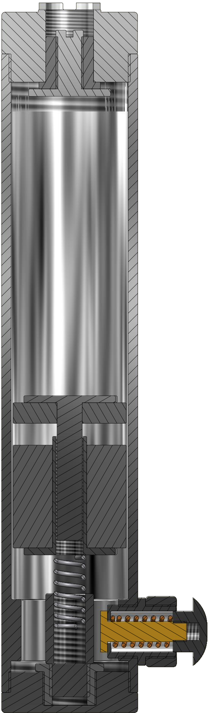
SECTION A-A SCALE 3 : 1
