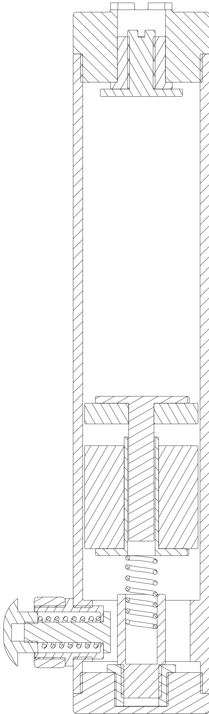
SECTION B-B SCALE 3 : 1
